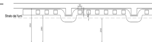
Dimensionamento canalizzazione per Compartimento 2
