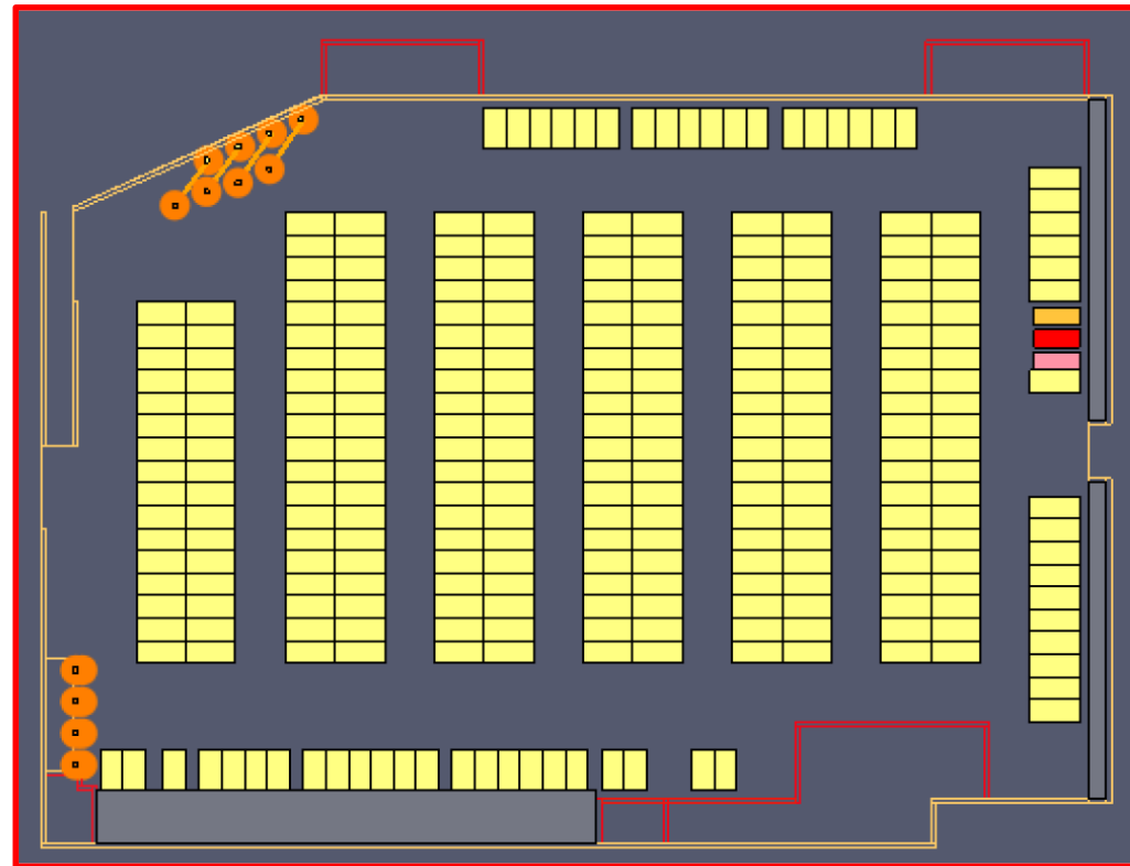
Posizionamento impianto di estrazione, comp. 2 (P-2)
