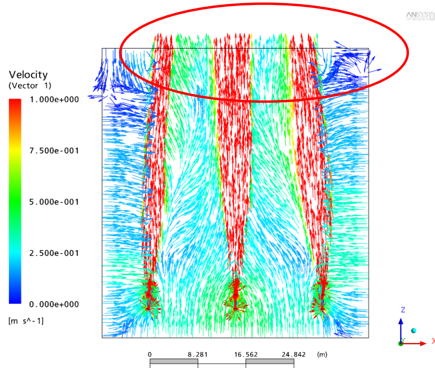
Getti dei ventilatori separati
