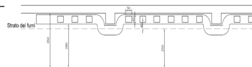
Dimensionamento canalizzazione per Compartimento 2
